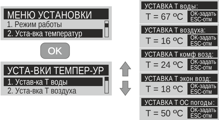
Рисунок 16 Установка температурных параметров
