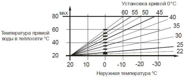
Рисунок 15 Отопительная кривая прибора. Вертикальная шкала – температура теплоносителя, горизонтальная - температура наружного воздуха.
